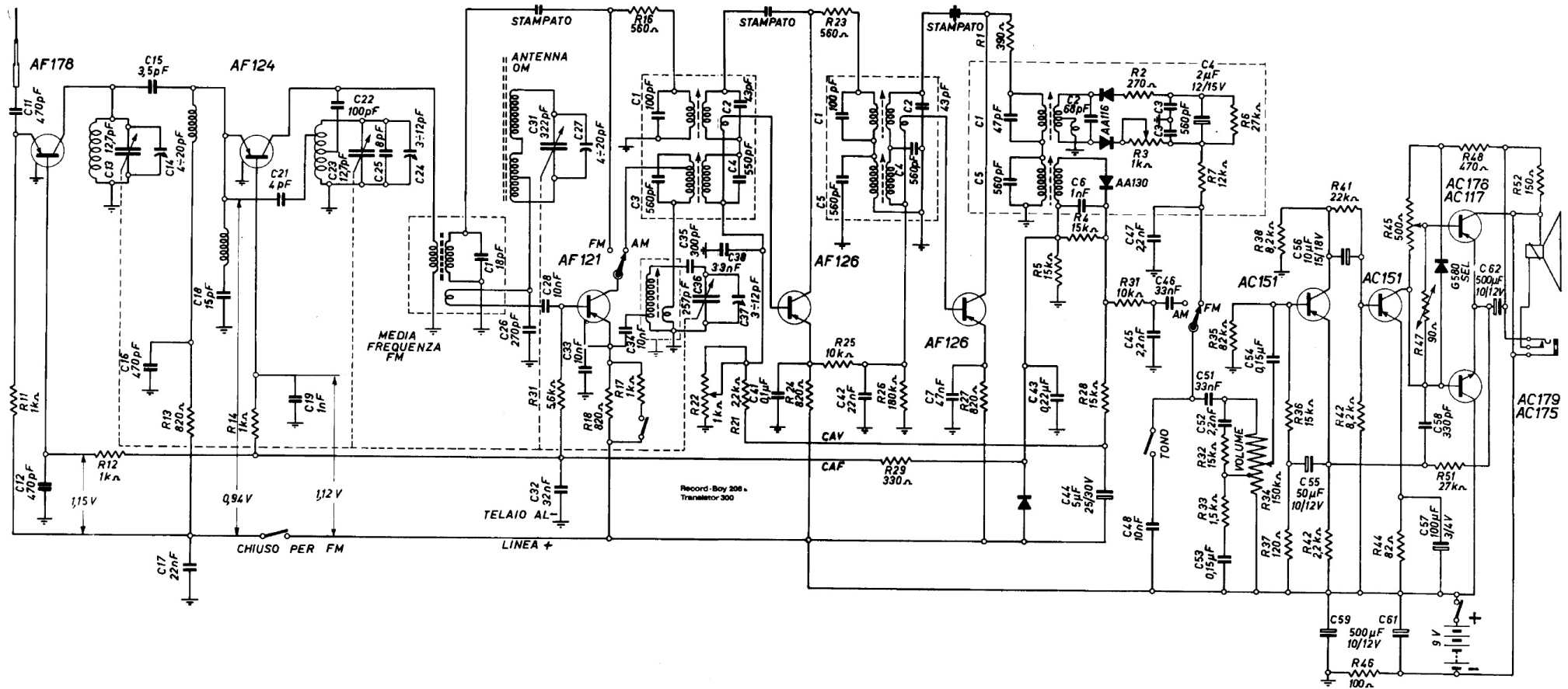
GRUNDIG - Mod. Record Boy 206 a e Transistor 300 - Onde medie da 510 a 1620 kc/s. Modulazione di frequenza da 87 a 108 megacicli. Media frequenza AM a 460 kc/s. Media Frequenza FM a 10,7 megacicli. Potenza d'uscita 1 watt. (V. retro circuiti stampati).
